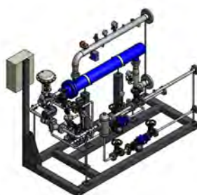
Gruppo Package Scambiatore a Fascio tubiero per Produzione Acqua Calda da Vapore a 7 Bar
