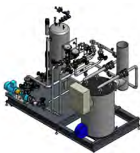
Gruppi Olio Diatermico con Sistema di Espansione Pressurizzato
